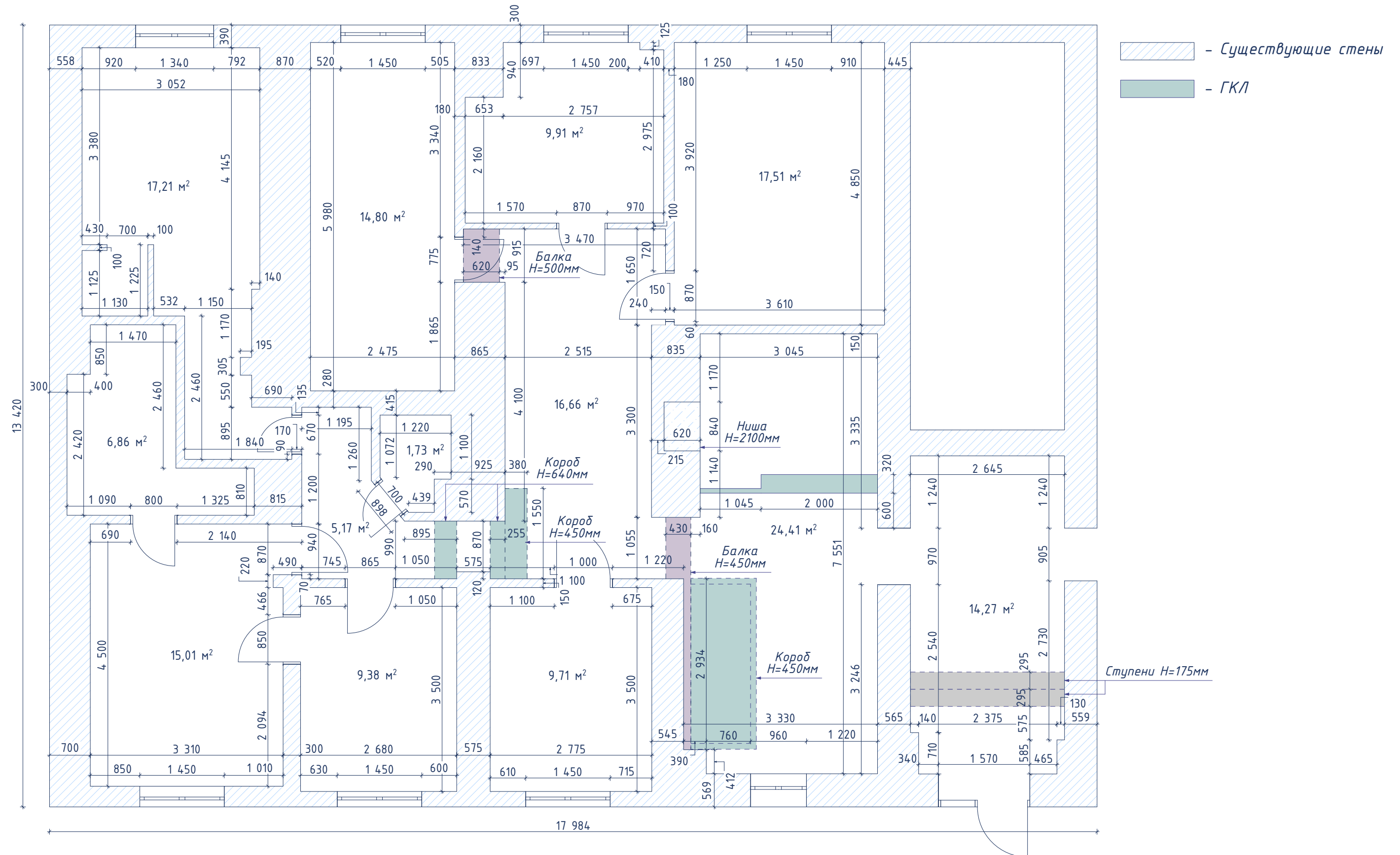
План левого крыла медицинского центра после перепланировки
